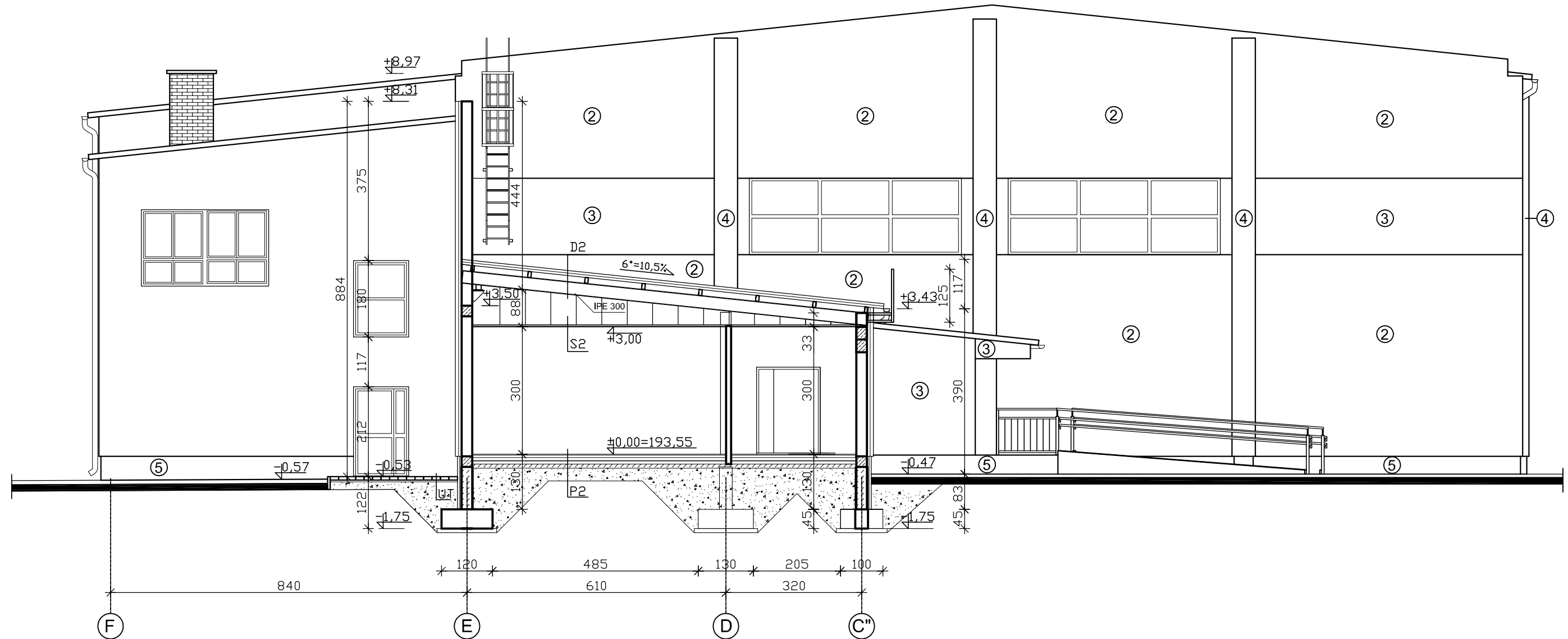
PRZEKRÓJ C-C SKALA 1:100
